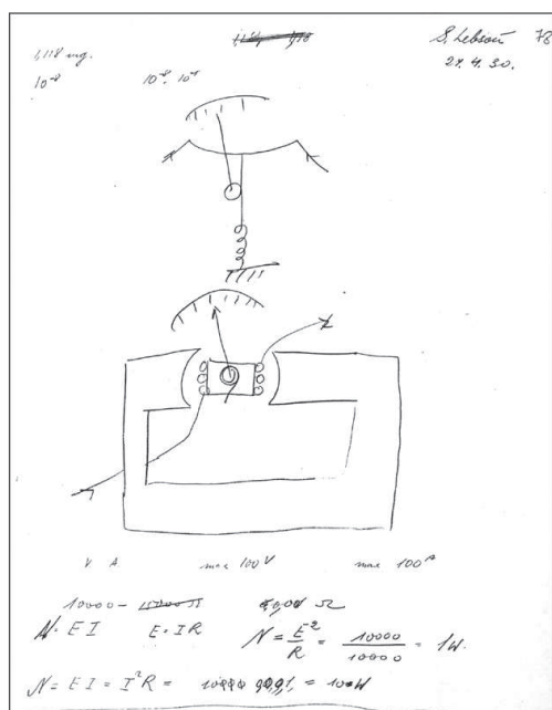
Rysunki Stefana Lebsona wyjaśniające działanie miernika magnetoelektrycznego na egzaminie 27.04.1930 roku – półdyplom
